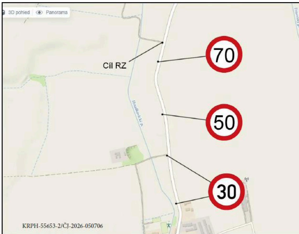
Situační schéma s vyznačeným umístěním přechodného dopravního značení
